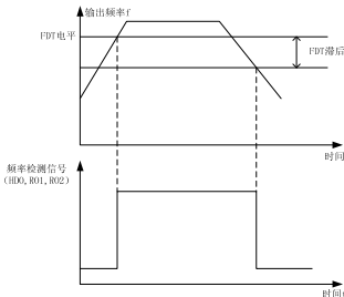
图 6-19 FDT 电平示意图
