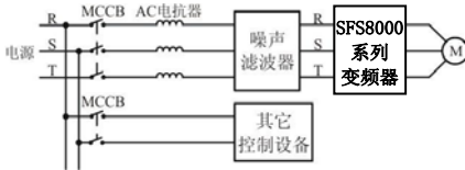
图 4-5 主回路电源侧连接图
