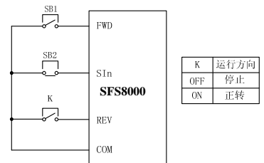
图 6-11 三线式运转模式 1 示意图
