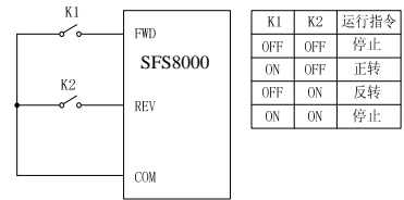
图 6-9 两线式运转模式 1 示意图
