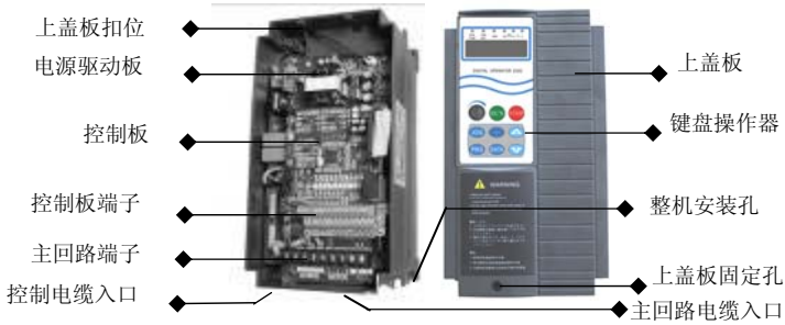
图 1-2 变频器各部分名称示意图
