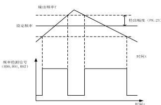
图 6-20 频率到达检出幅值示意图
