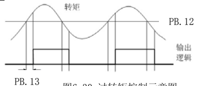
图6-30 过转矩控制示意图
