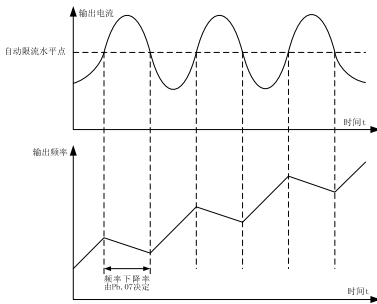
图 6-29 限流保护功能示意图
