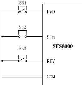
图6-12 三线式运转模式2示意图
