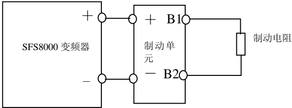
图 2.2 制动单元的连接
