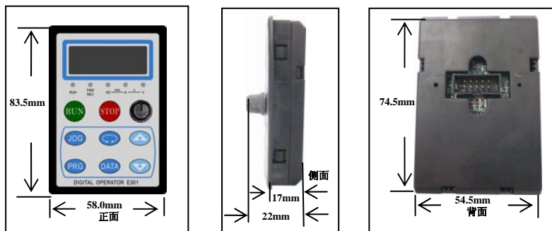
图 1.5.3-2 键盘操作器外形及安装尺寸图
