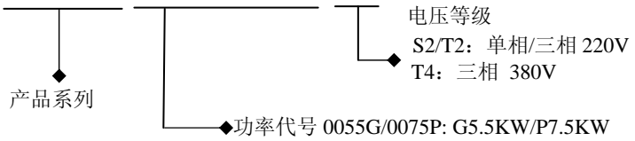
图 1-1 变频器铭牌说明
