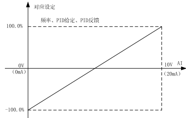
图 6-13 模拟给定与设定量的对应关系
