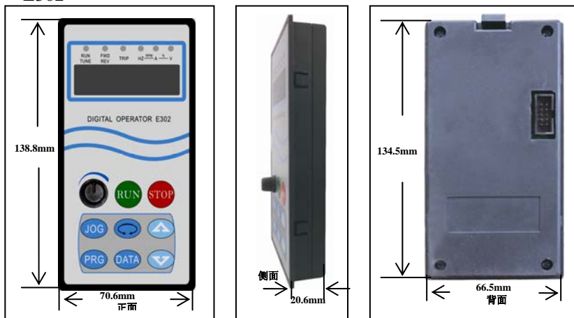
图 1.5.3-1 键盘操作器外形及安装尺寸图
