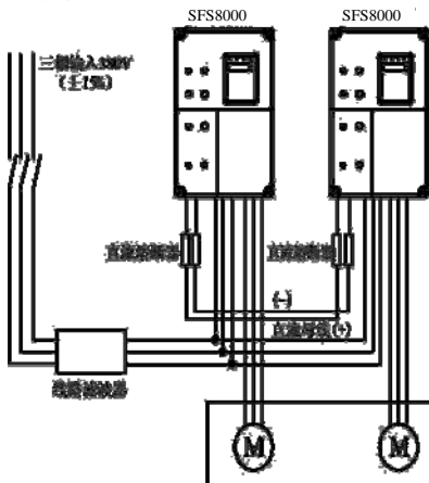
图 4-7 共直流母线的连接
