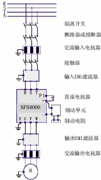
图 4-1 外围设备连接图
